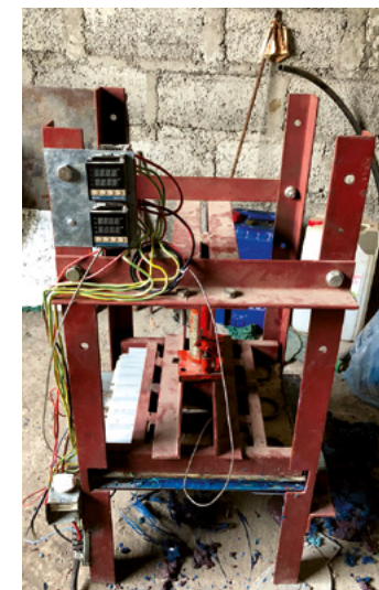
Presse chauffante pour fabriquer des panneaux à partir de déchets plastiques recyclés.
